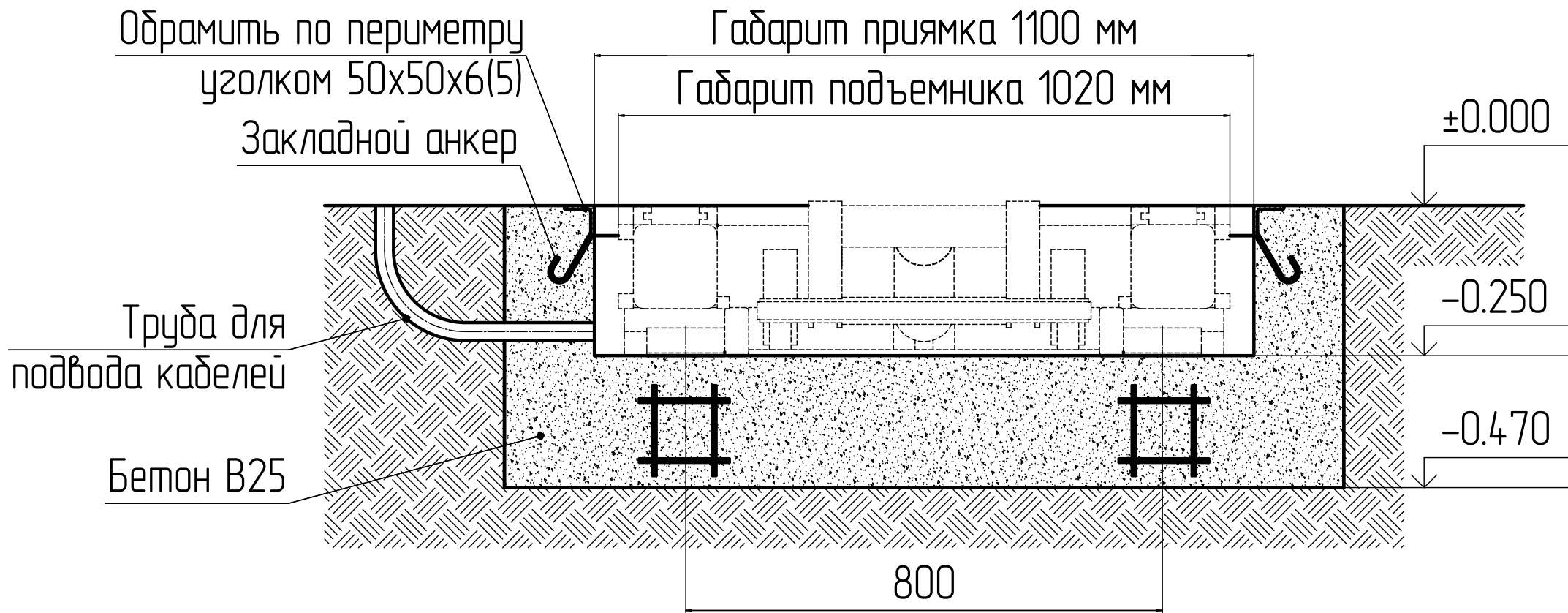
Рисунок 1 - Поперечное сечение
