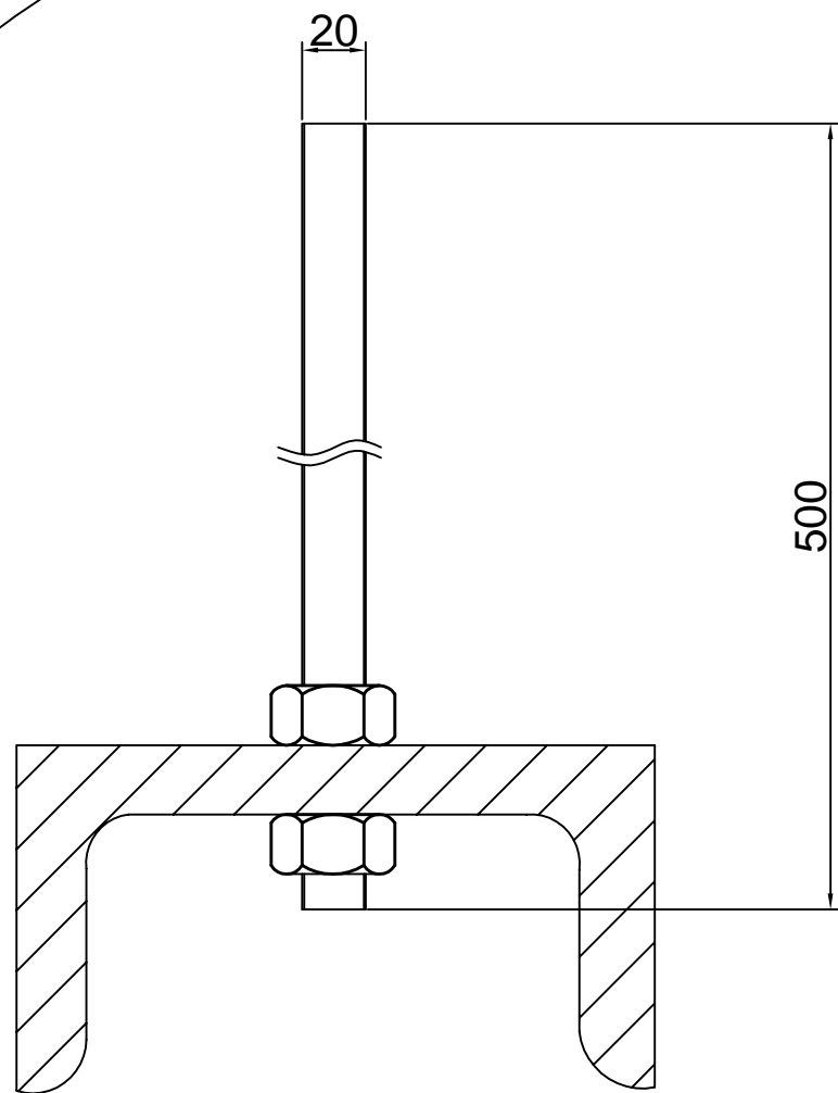
Закладная деталь: швеллер П200 со шпилькой М20
